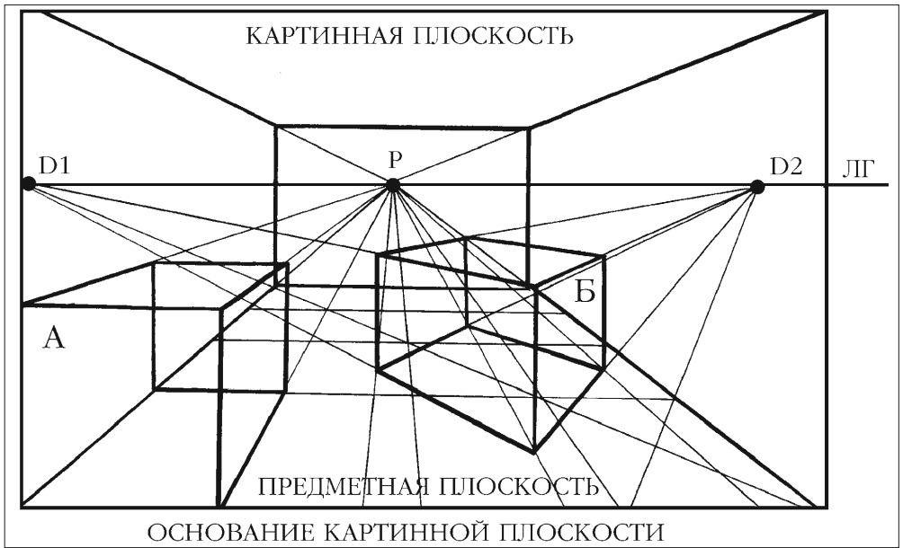
Схема перспективного построения с основными ее элементами
